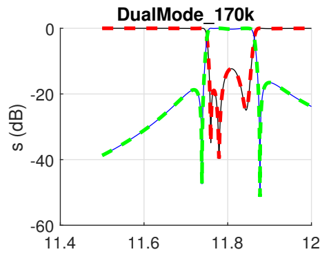
interp, Threshold=1.0e-05, snapshots=123288x34 Matlab - projekcja, Qsize=23
