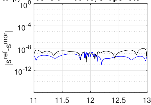
interp, Threshold=1.0e-05, snapshots=137892x54 Matlab - projekcja, Qsize=30
