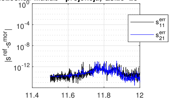
interp, Threshold=1.0e-05, snapshots=123288x34 Matlab - projekcja, Qsize=23
