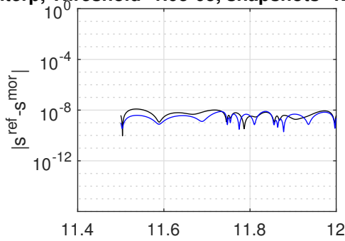
interp, Threshold=1.0e-05, snapshots=123288x34 Matlab - projekcja, Qsize=23
